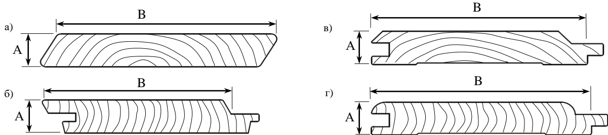
Рисунок 1: Профиль ФД: а) ФД1; б) ФД2; в) ФД3; г) ФД4. Тип соединения: ФД1 – внахлест; ФД2, ФД3, ФД4 – паз-гребень
